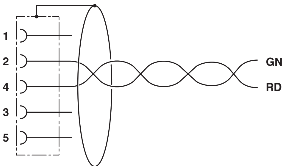
电路图
