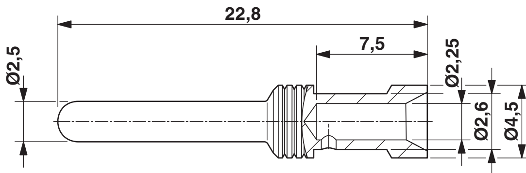
尺寸图
