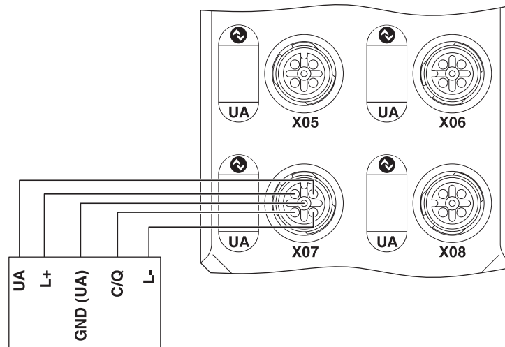
接线图
