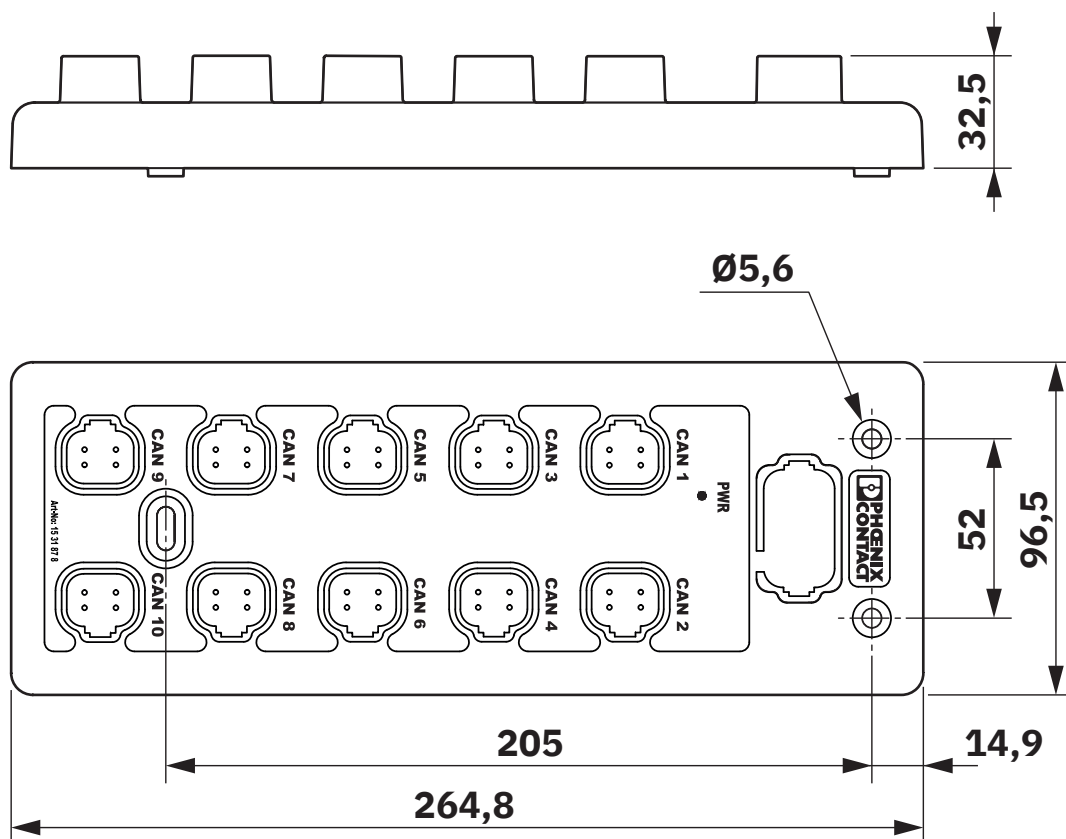
Dessin coté
