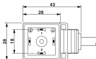
外形寸法
