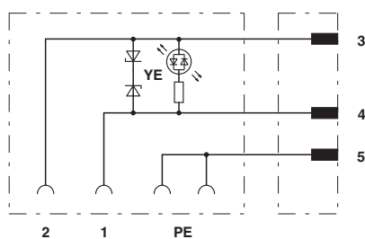
回路図
