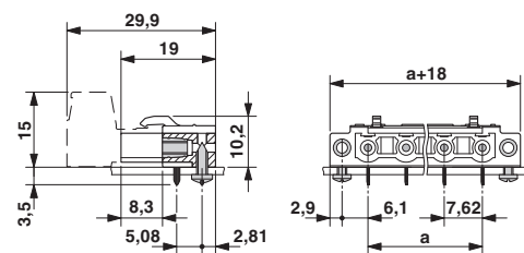
外形寸法
