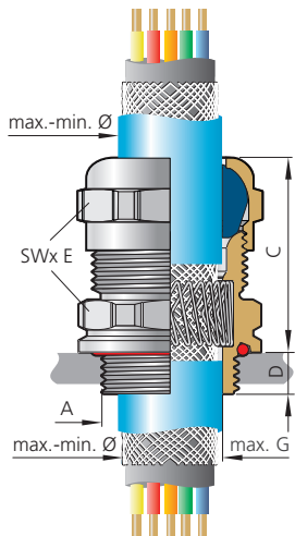
Abb. 4 – Variante B: durchgängiger Außenmantel Fig. 4 – Method B: continuous outer sheath
