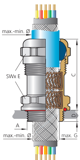
Abb. 3 – Variante A: abgesetzter Außenmantel Fig. 3 – Method A: offset outer sheath
