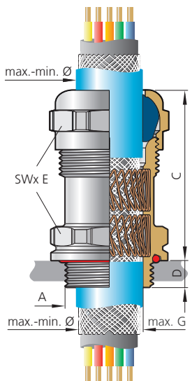
Abb. 4 – Variante B: durchgängiger Außenmantel Fig. 4 – Method B: continuous outer sheath
