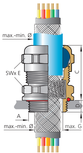
Abb. 3 – Variante A: abgesetzter Außenmantel Fig. 3 – Method A: offset outer sheath
