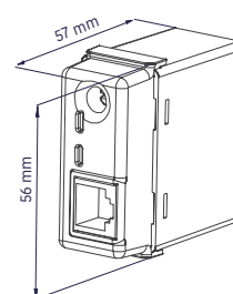
Ethernet module
