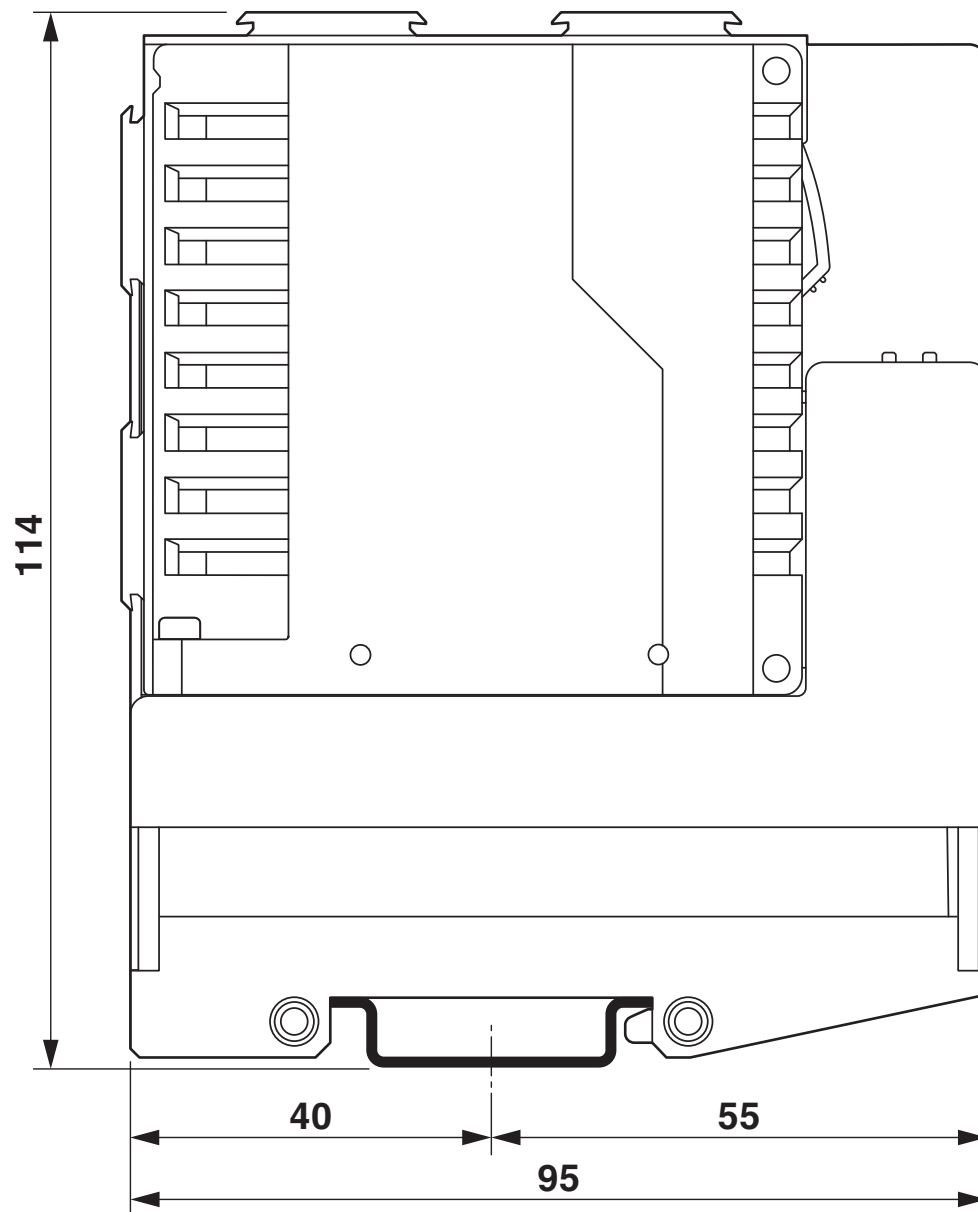
Maßzeichnung
