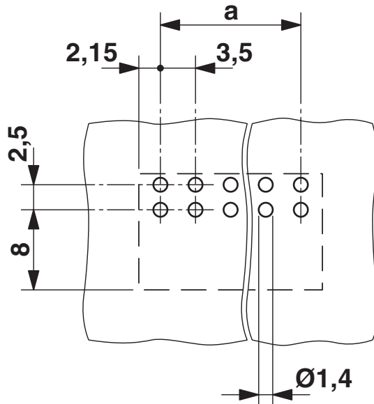
Bohrplan/Lötpadgeometrie
