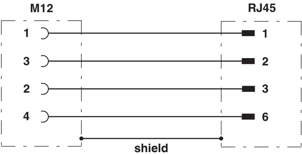
电路图
