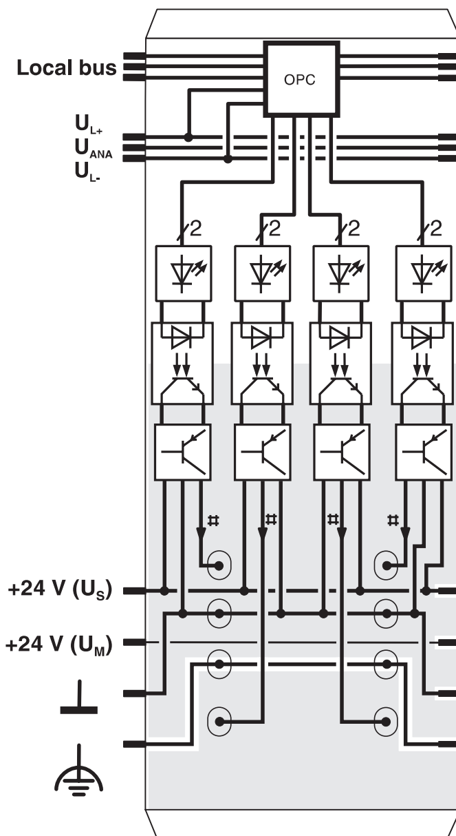
结构框图
