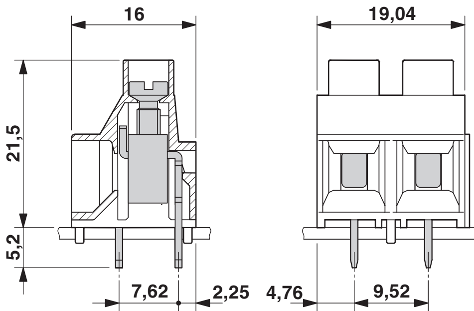
尺寸图
