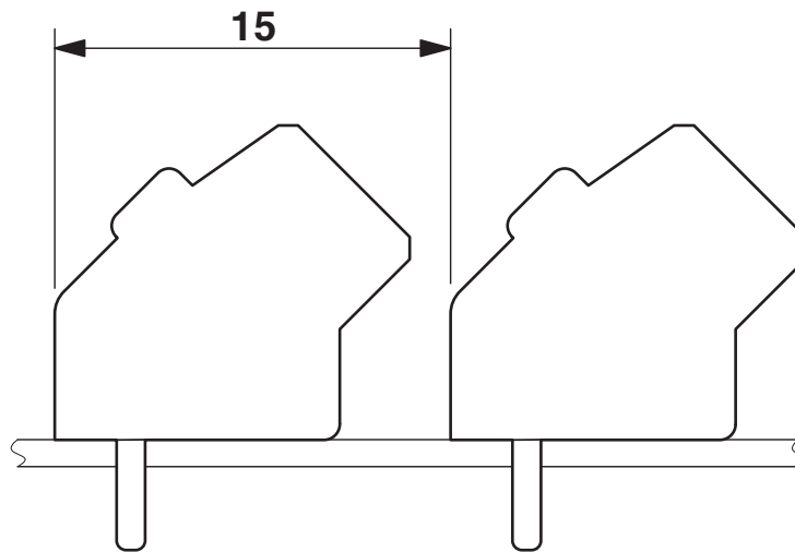
尺寸图
