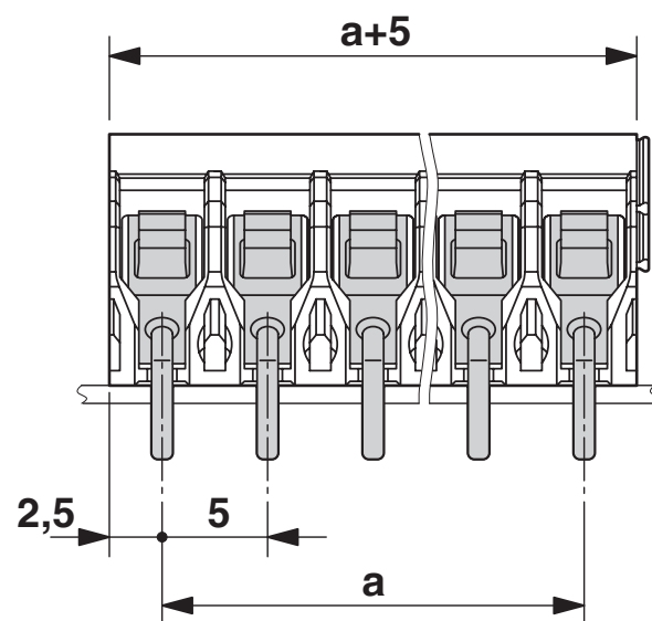
尺寸图
