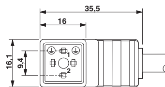
外形寸法
