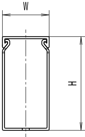
Montagezustand mit Deckel/ Assembly condition with cover
