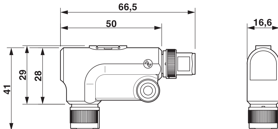
尺寸图
