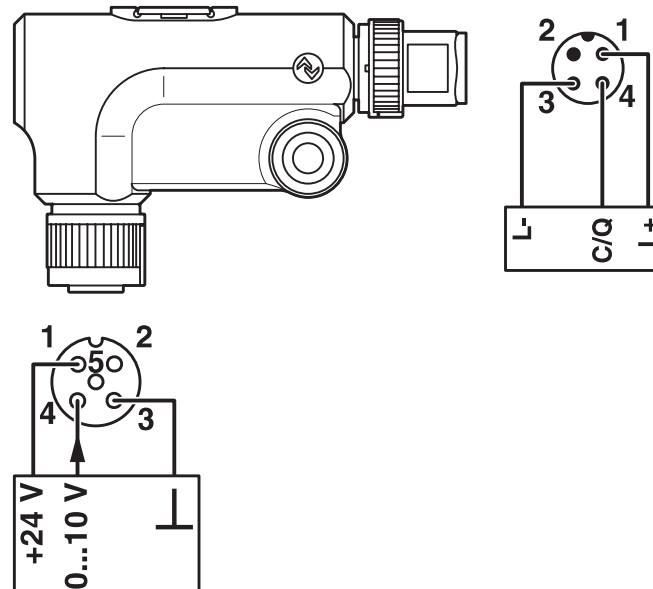
接线图
