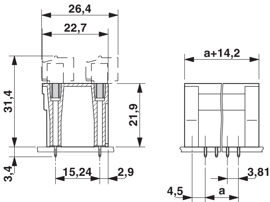
尺寸图
