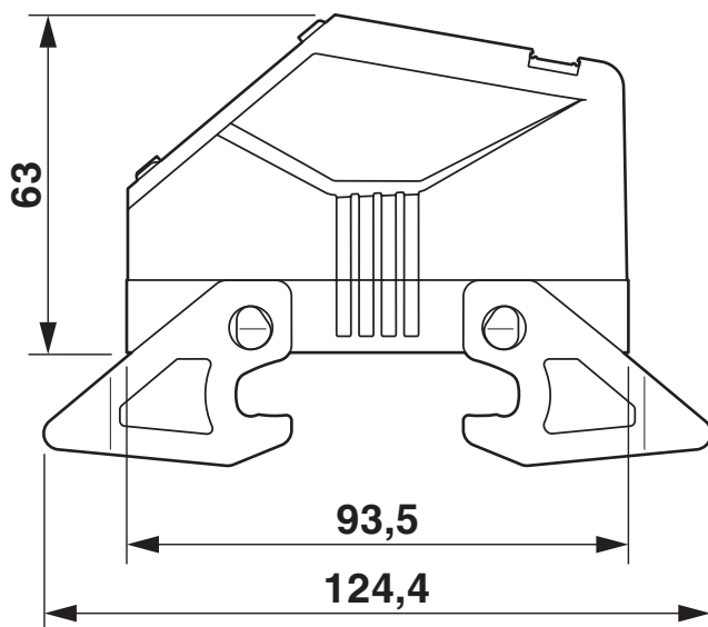
尺寸图
