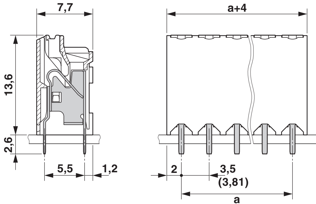
尺寸图
