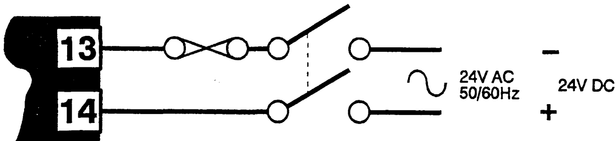
Abb.: 3 - 7 24 V AC / DC Spannungsversorgung
