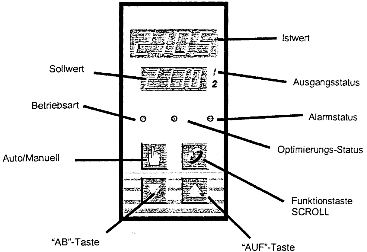
Abb.: 2 - 1 Anzeige und Bedienung
