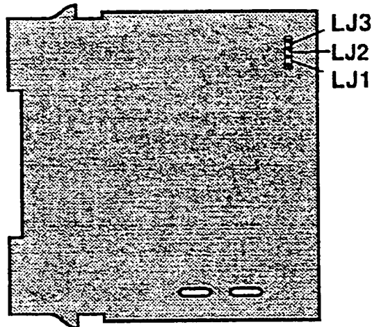
Abb.: 7-4 CPU Platine Eingangswahl
