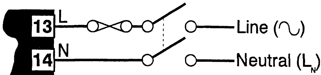
Abb.: 3 - 6 Netzanschluß
