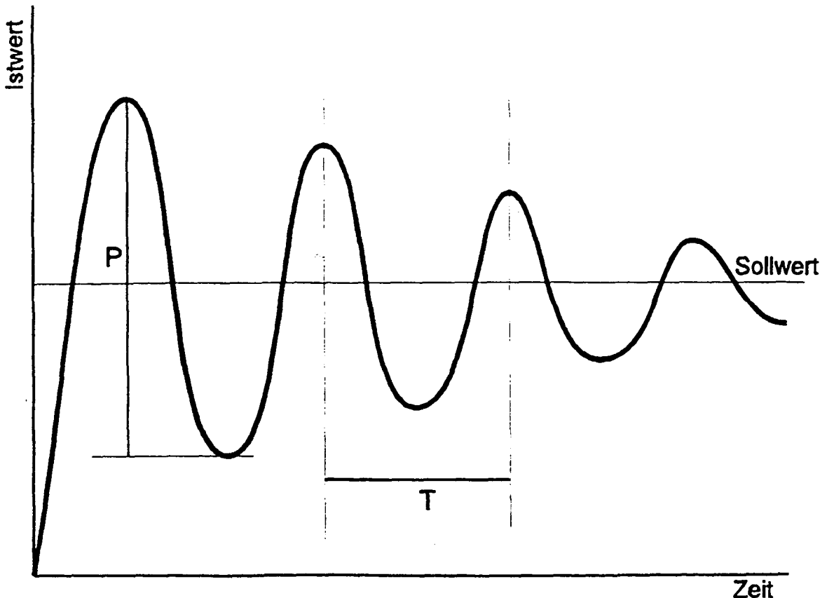
Abb.: 4-4 Abstimmen eines Zweipunktreglers
