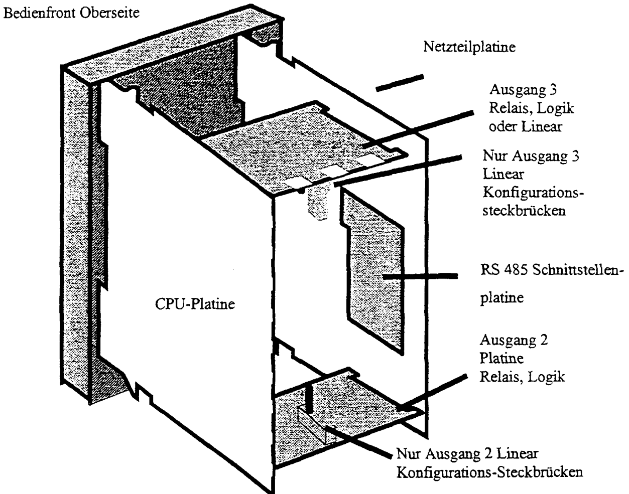
Abb.: 7-1 Regler - Platinenanordnung
