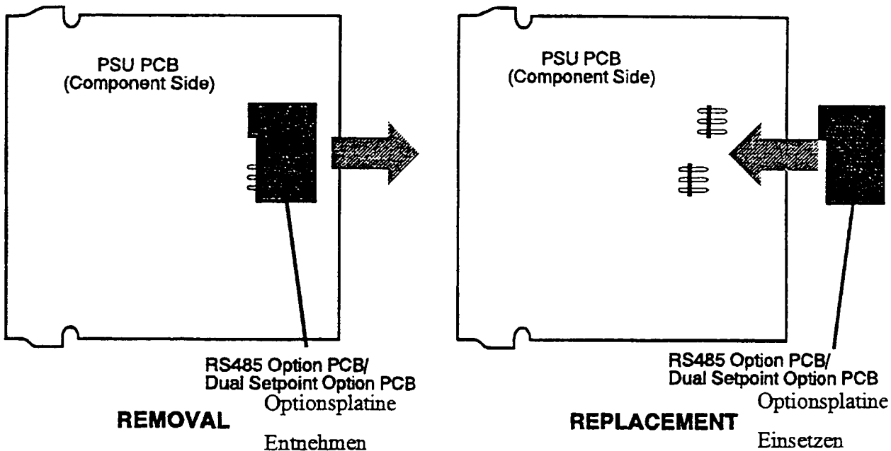
Abb.: 7-3 Auswechslern der Optionsplatine
