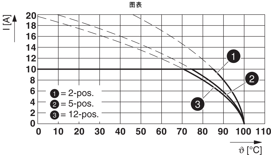
型号 : FKCN 2,5/...-ST , 带MDSTBA 2,5/...-G
