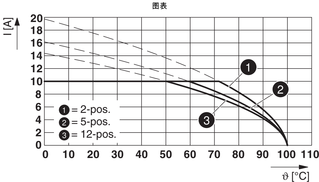
型号 : FKCN 2,5/...-ST , 带MDSTBV 2,5/...-G
