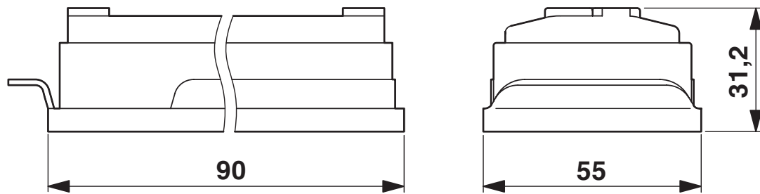
尺寸图
