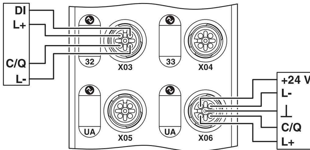
接线图
