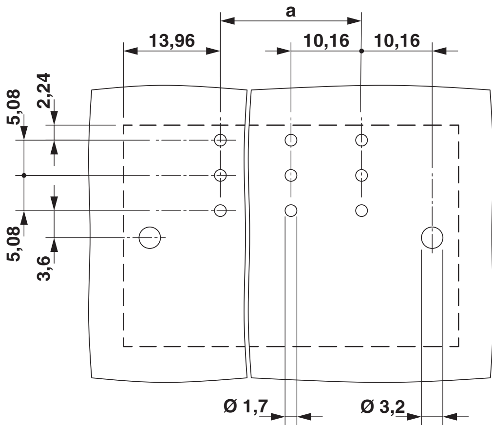
开孔图/焊盘环宽
