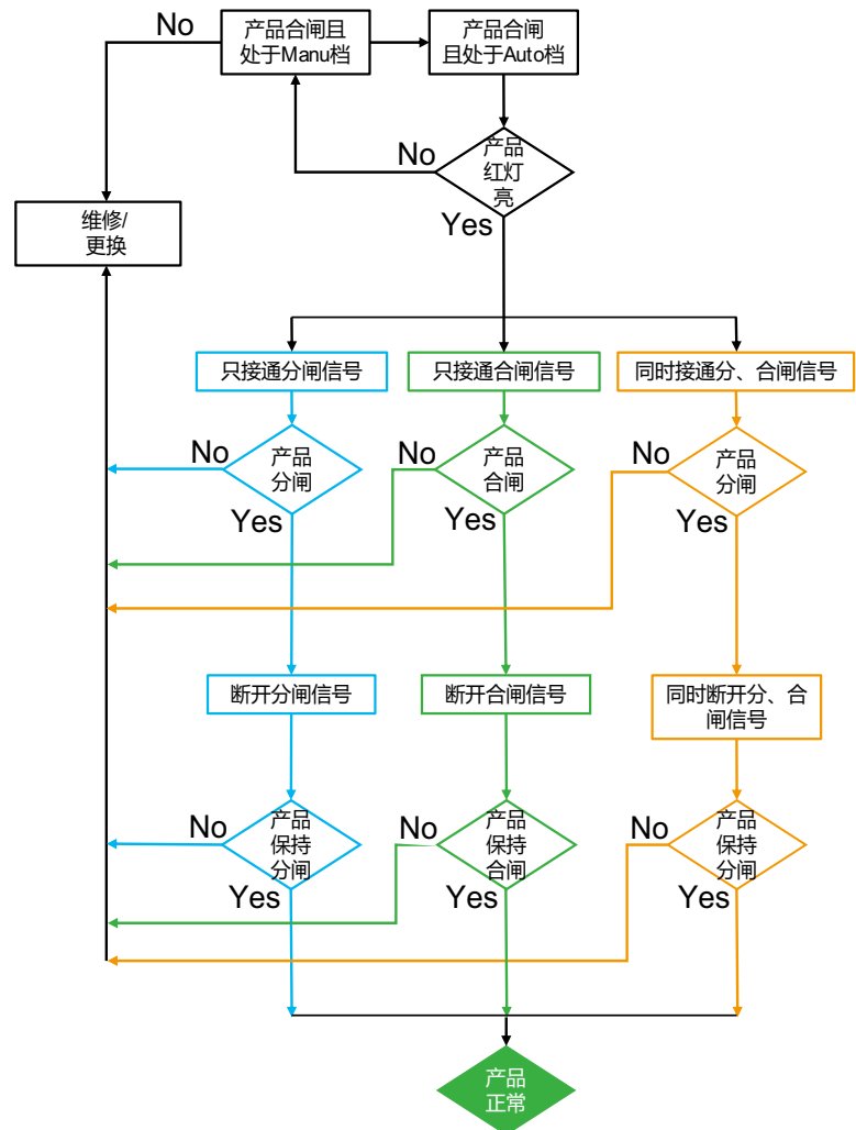
RCA逻辑图
