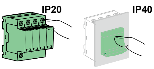
安装在35mm标准导轨上
