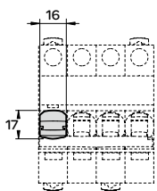
挂锁附件
