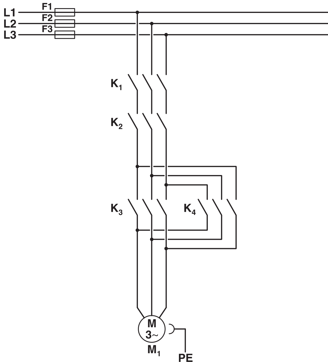
电路图
