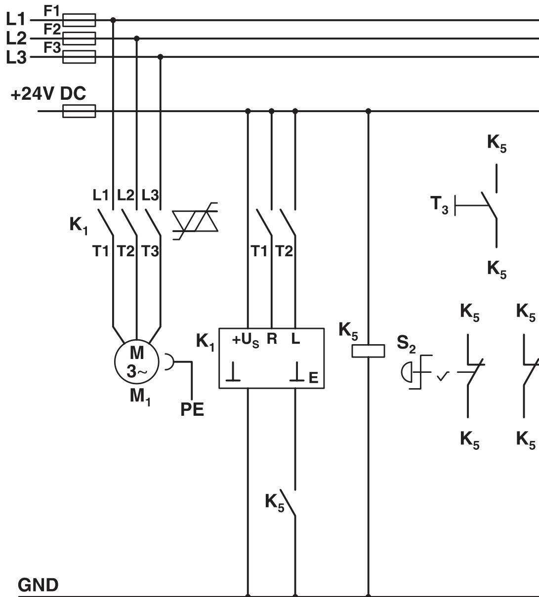
电路图
