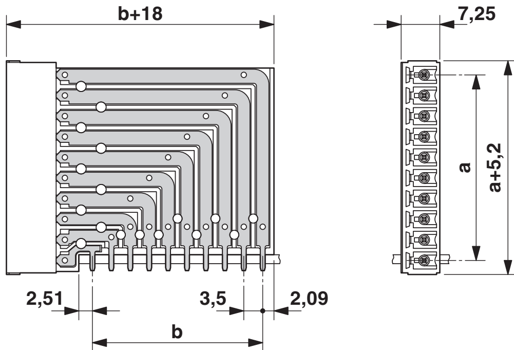
尺寸图
