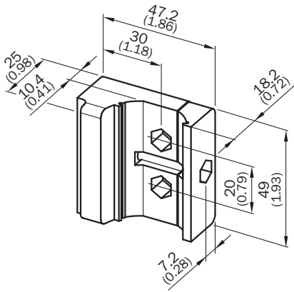
尺寸圖 (尺寸 (mm))
