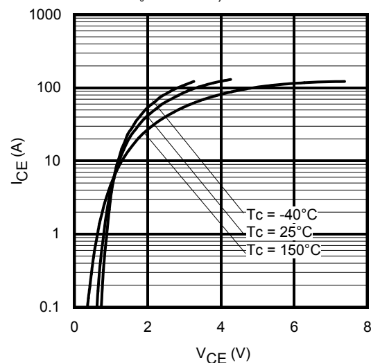
Fig. 5 - Typ. IGBT Saturation Voltage V_{\text{GE}} = 15\text{V} ; t_p = 20\mu\text{s}
