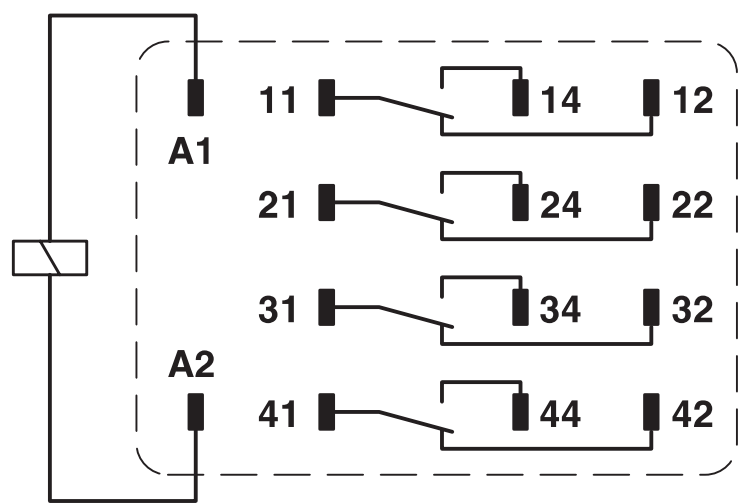
电路图
