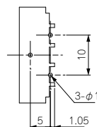
BCR20V4外観寸法図
