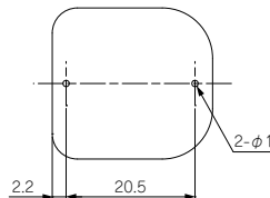
BCR20H5外観寸法図
