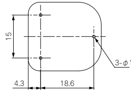
BCR20H4外観寸法図
