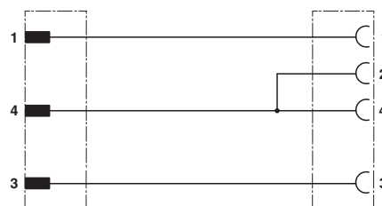
回路図
