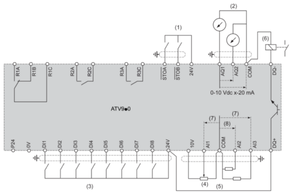
控制块接线图
