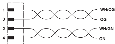
回路図
