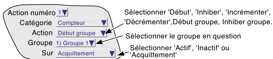
Figure 4.7.7 Actions sur les compteurs (action groupe)
