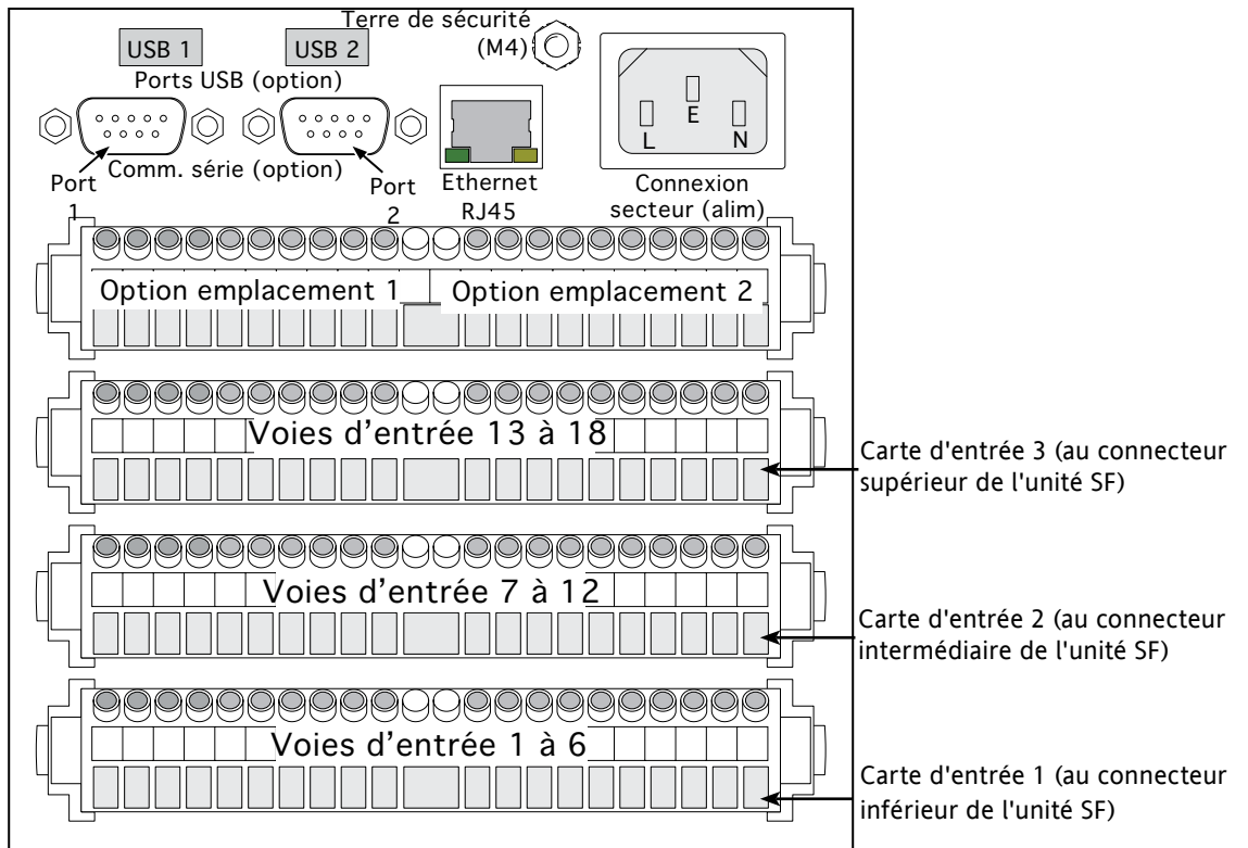
b. Enregistreur
