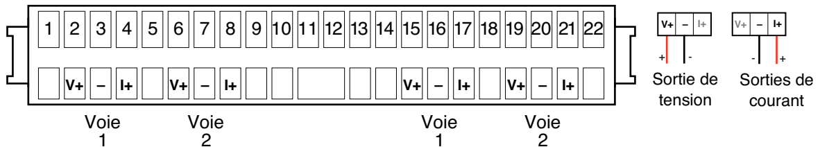
Figure 2.2.1d Câblage des options page 1
