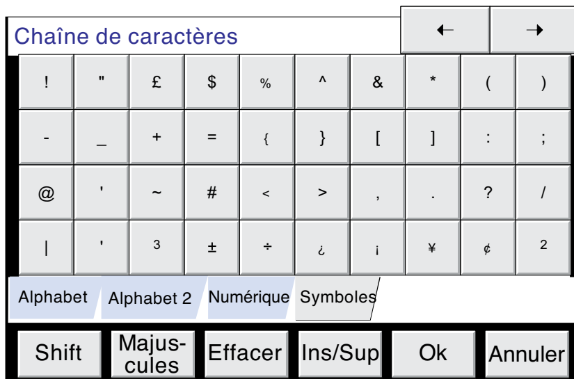
Figure 3.3.1c Autres claviers
