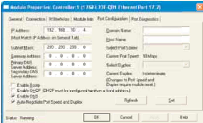
Figure 4.3.21i Propriétés du module
