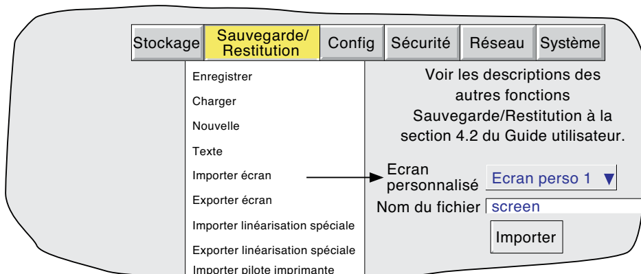
Figure 7.1.2 Menu Sauvegarde/Restitution (Importer écran)
