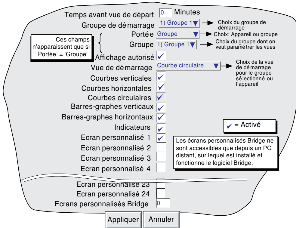
Figure 7.1.1 Menu de configuration des vues
