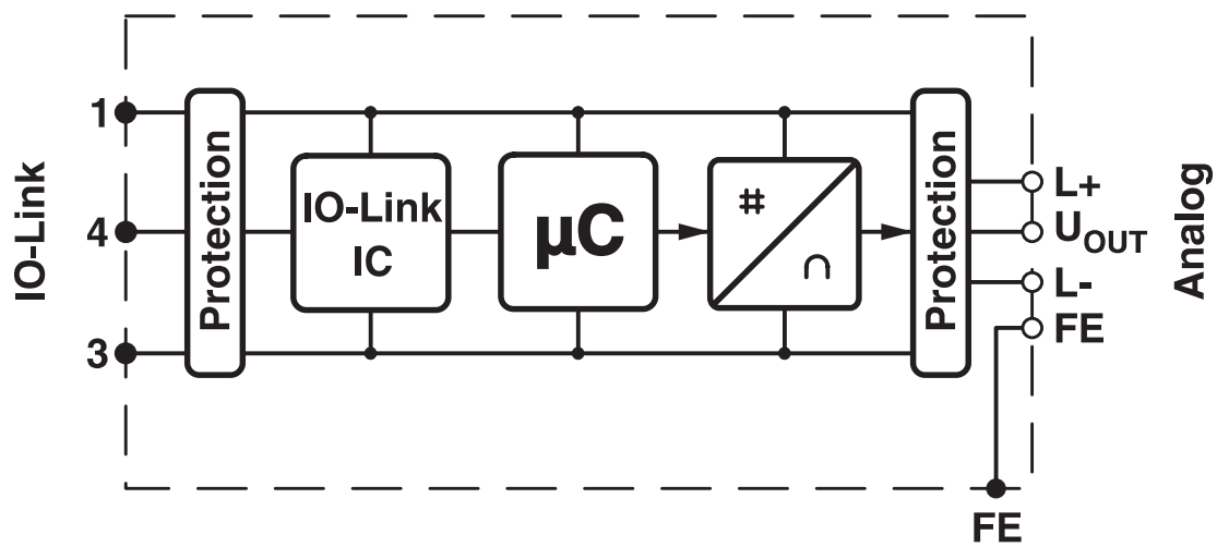
结构框图
