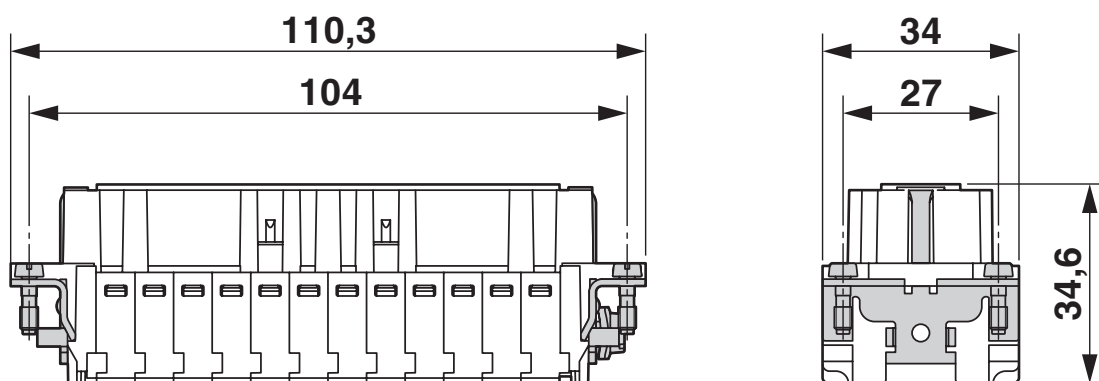
尺寸图
