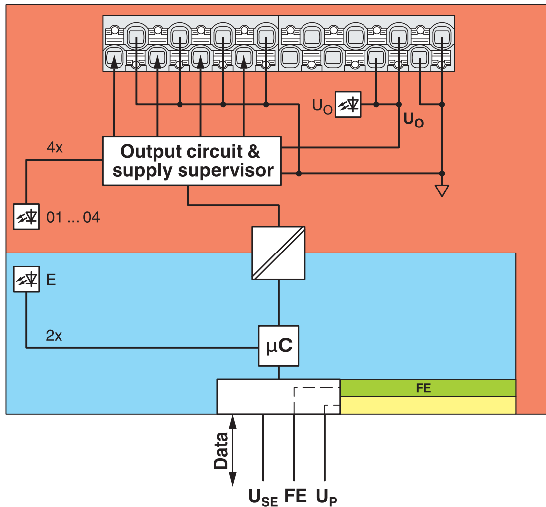
结构框图
