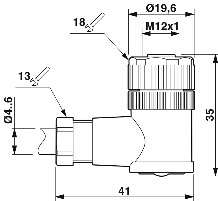
尺寸图
