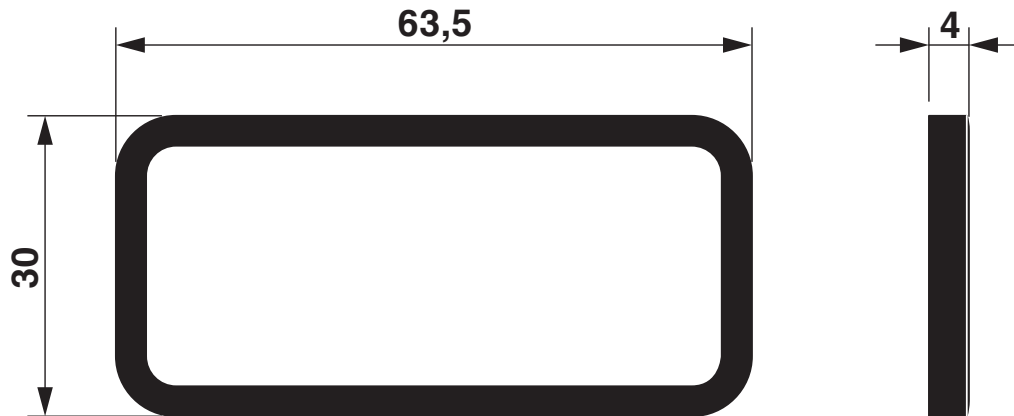
尺寸图
