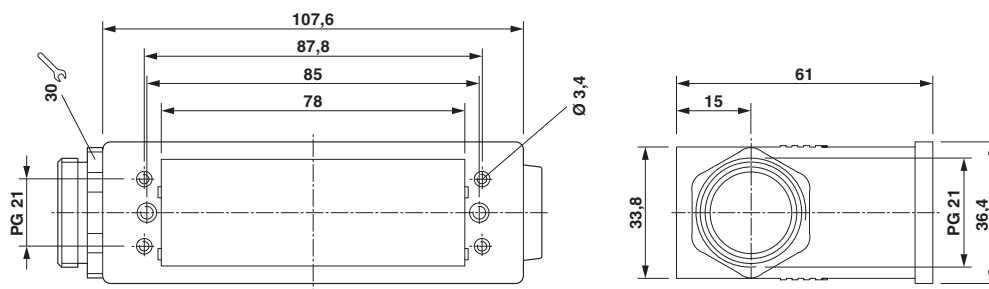
尺寸图
