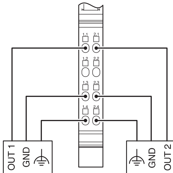
接线图
