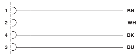
M12ソケットのコンタクト配列
