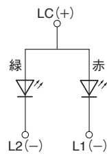
超高輝度LED(輝度レベル2) 周囲温度 Ta=25°C
