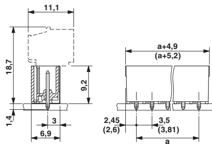
外形寸法
