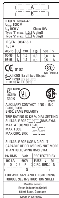
Abbildung/Figure 2: Typenschild/Rating plate ZB150/XTOB...GC1
