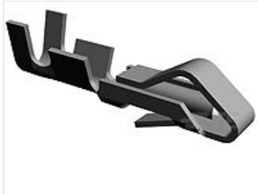
TE Part #640252-2 SL-156 RECEPTACLE
