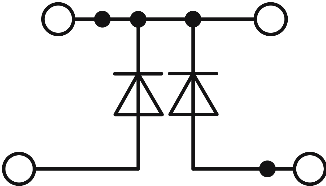
电路图
