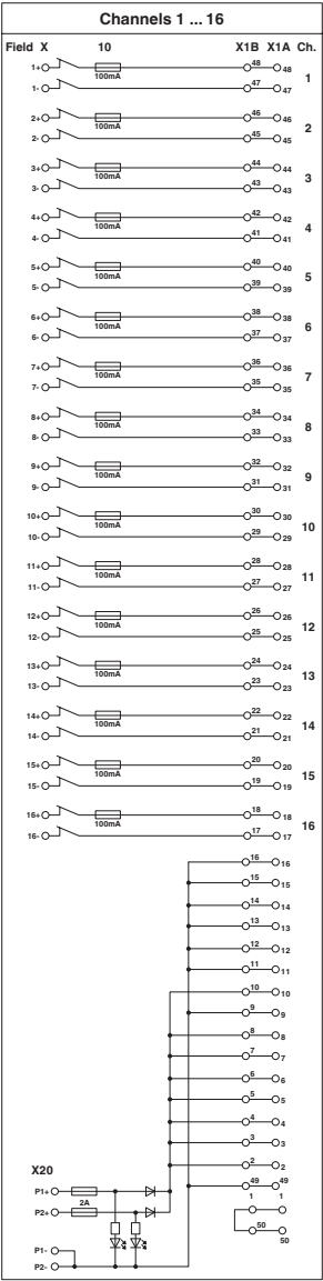
电路图
